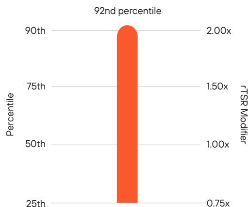
rTSR Modifier
